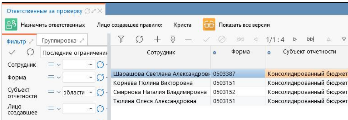
Рисунок 6 – Внешний вид интерфейса «Ответственные за проверку»
